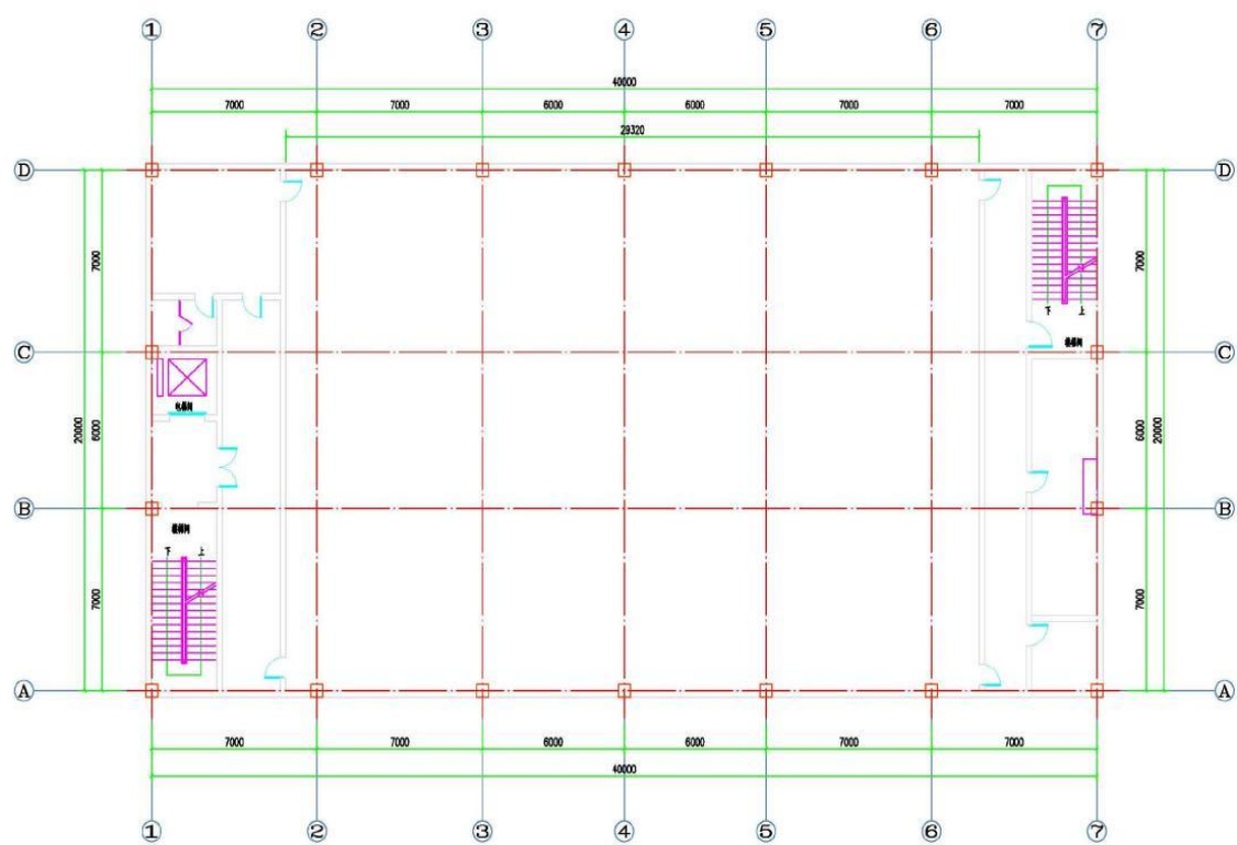
中药制剂楼4楼建筑平面图
